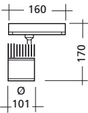
Technische Zeichnung / Technical drawing (mm):
