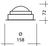
Technische Zeichnung / Technical drawing (mm):
