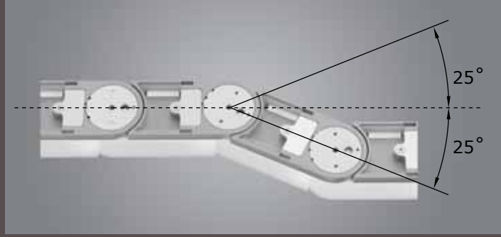
Modül mafsals hareketi / Rotating pivot joints
